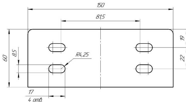
Рисунок 6 - Кронштейн светильника (ДСП36-110-270 Вт).
