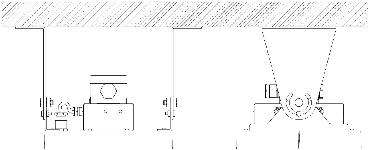
Рисунок 4 - Схема установки светильника (110-270 Вт) на потолок (стену).
