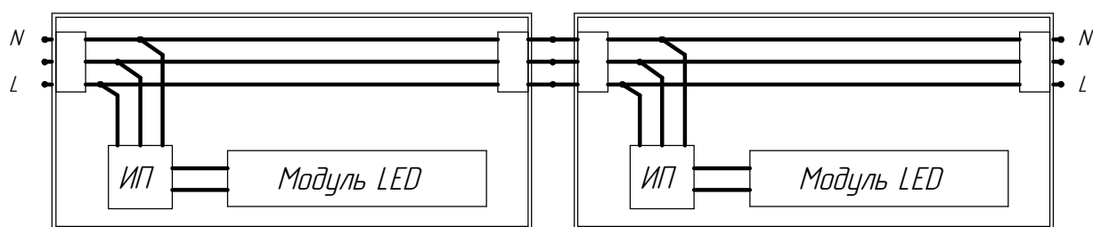
Рисунок 4 - Схема сквозной проводки (ДПО48-XX-1XX)
