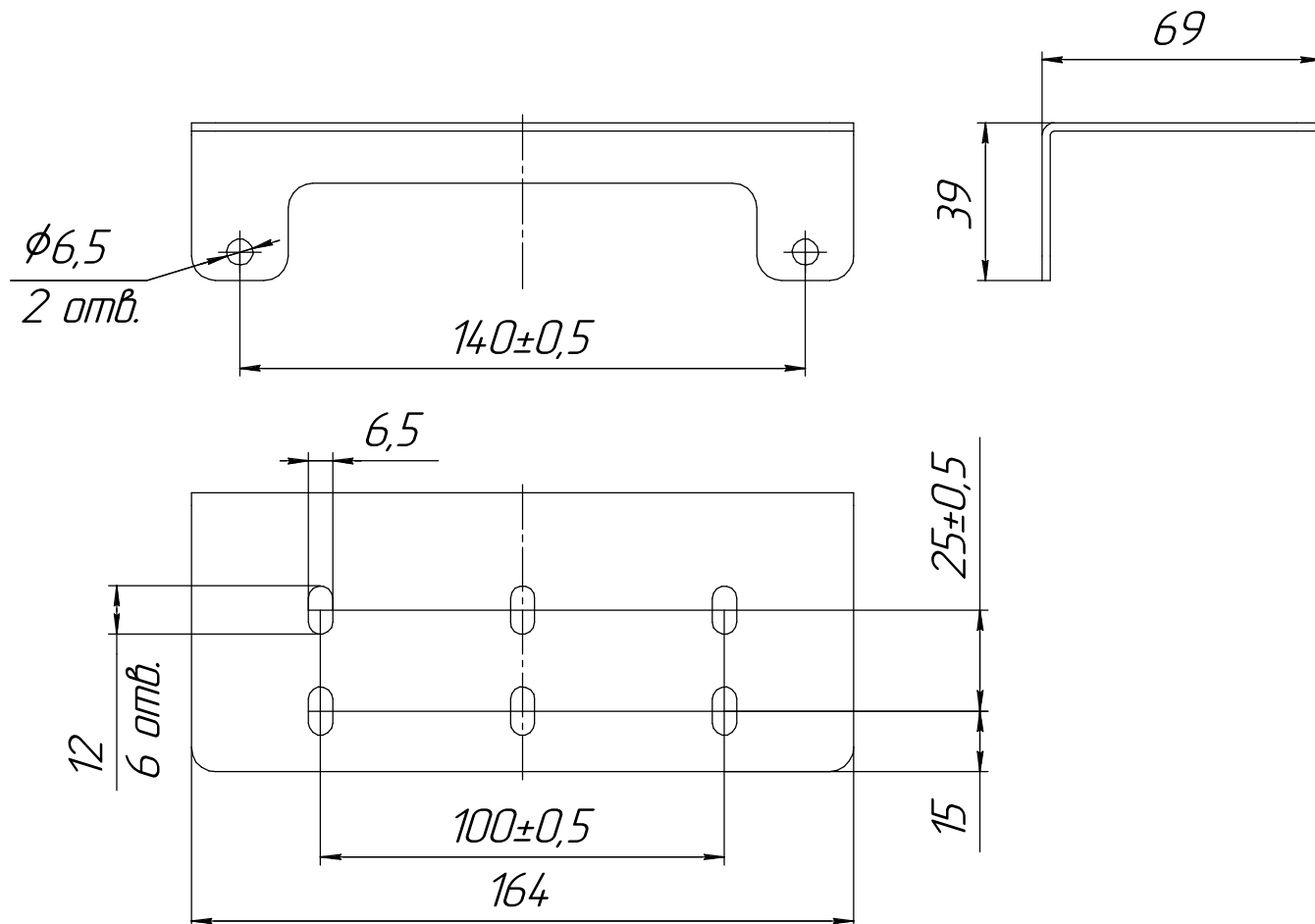
Рисунок 6 - Кронштейн 734313040.
