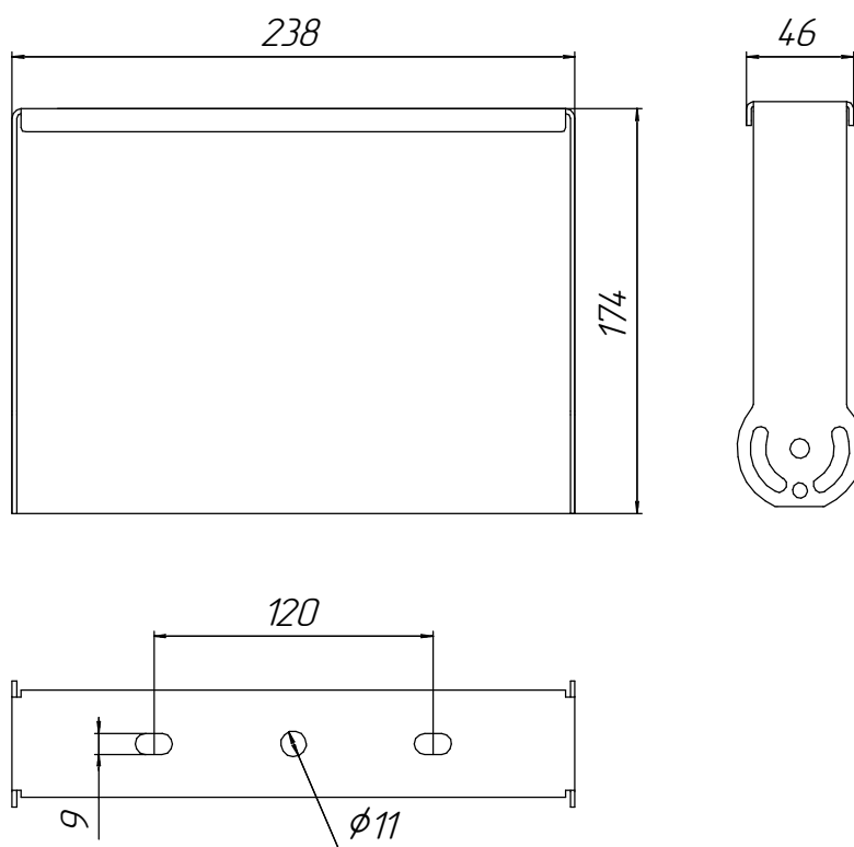
Рисунок 10 - Лира 745361027.
