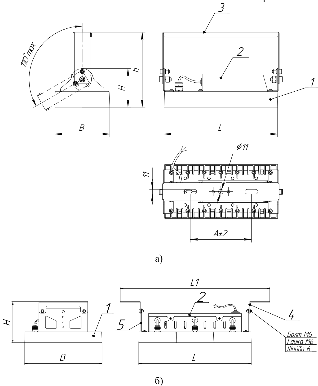
Рисунок 1 - Внешний вид и габариты светильников серии ДСП19 Quant
