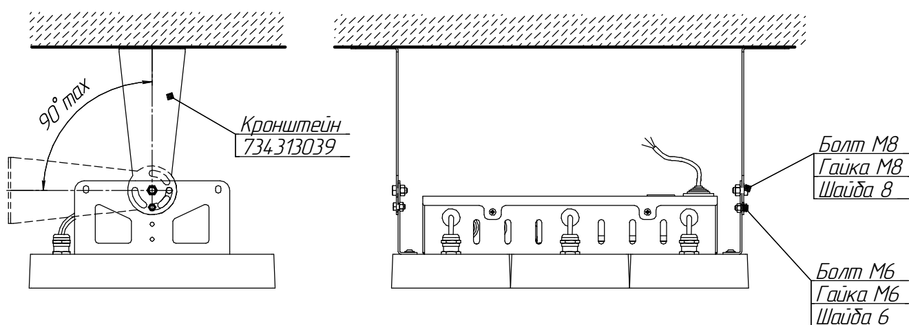
Рисунок 7 - Схема установки светильника (110-270 Вт) на потолок (стену) с помощью кронштейна 734313039.
