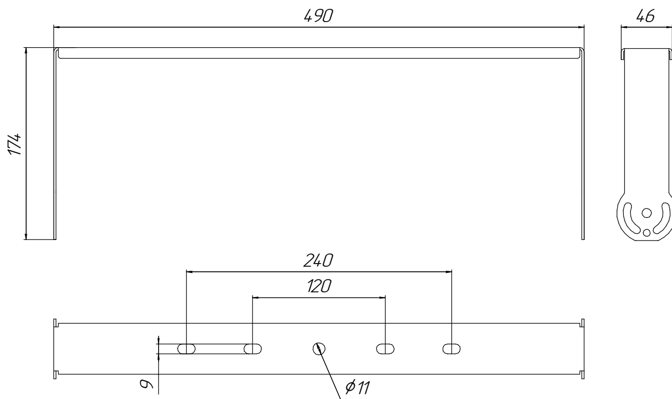
Рисунок 11 - Лира 745361027-01.
