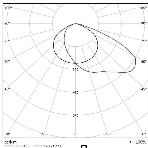
Рисунок 4 - Тип КСС светильника
