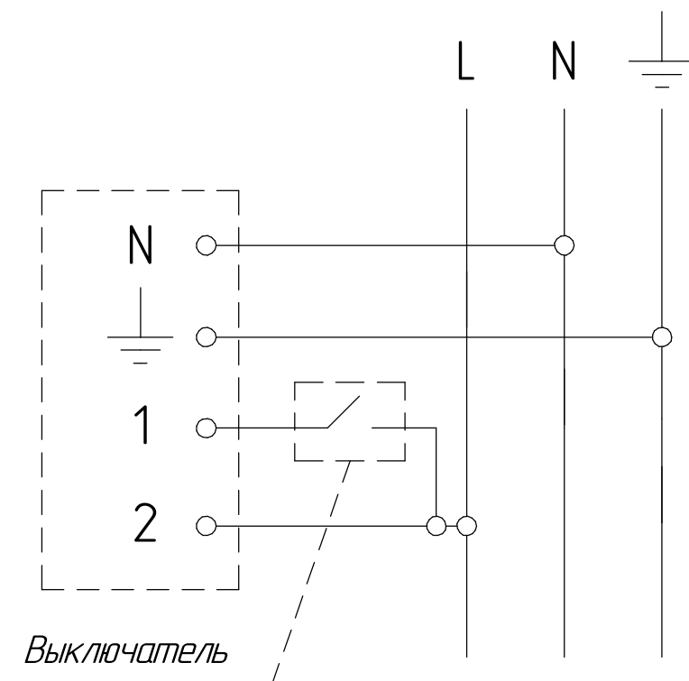
Рисунок 8 - Схема подключения светильников с БАП к сети
