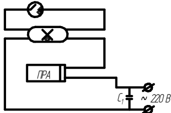
Рисунок 2. Схема электрическая принципиальная.
