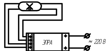
Рисунок 5. Схема электрическая с электронным ПРА.
