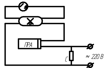
Рисунок 3. Схема электрическая принципиальная с параллельной компенсацией.
