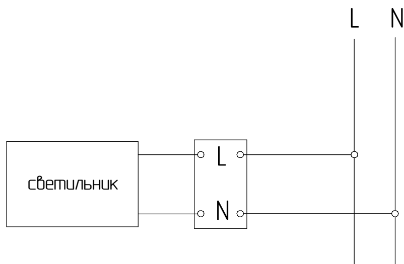
Рисунок 5 - Схема подключения светильника к сети
