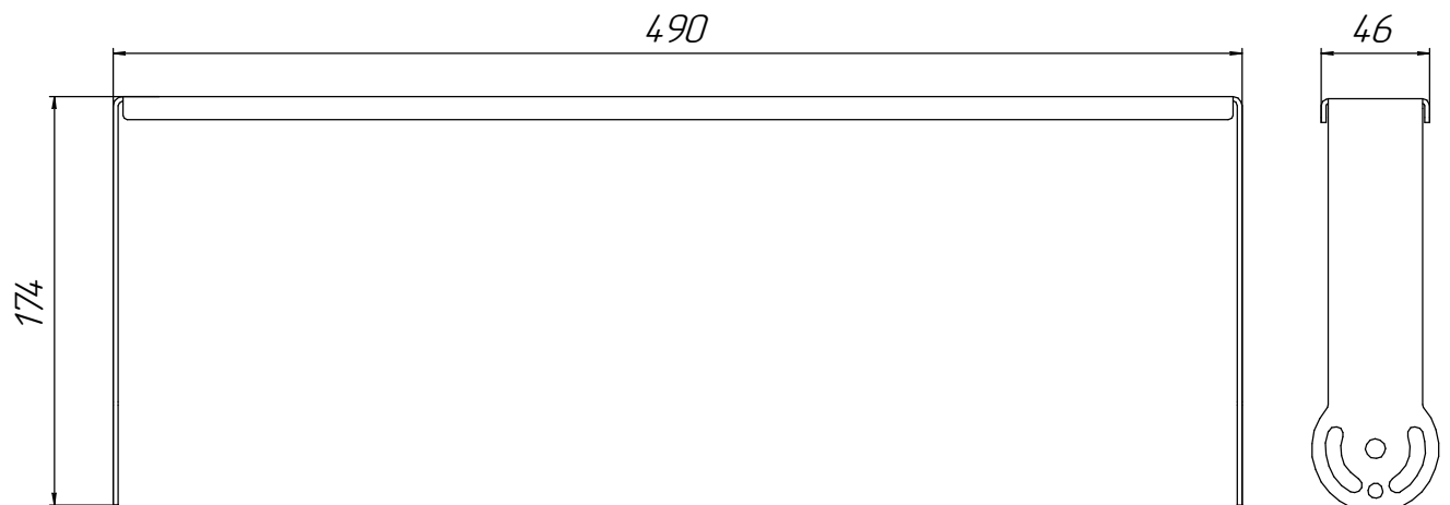
Рисунок 11 - Ли́ра 745361027-01.
