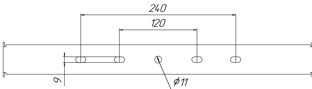
Рисунок 12 - Ли́ра 745361027-02.
