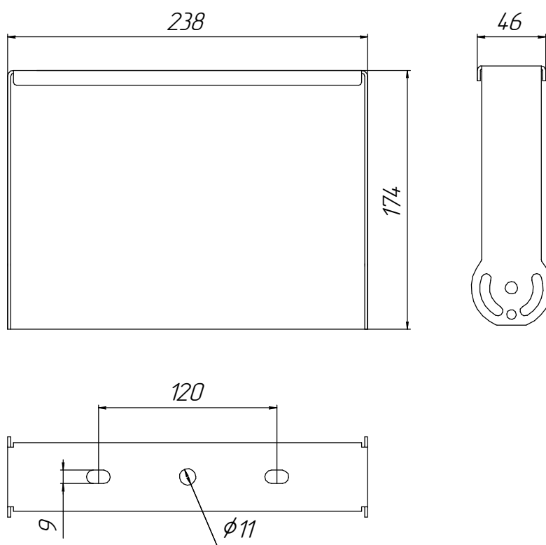
Рисунок 10 - Лира 745361027.
