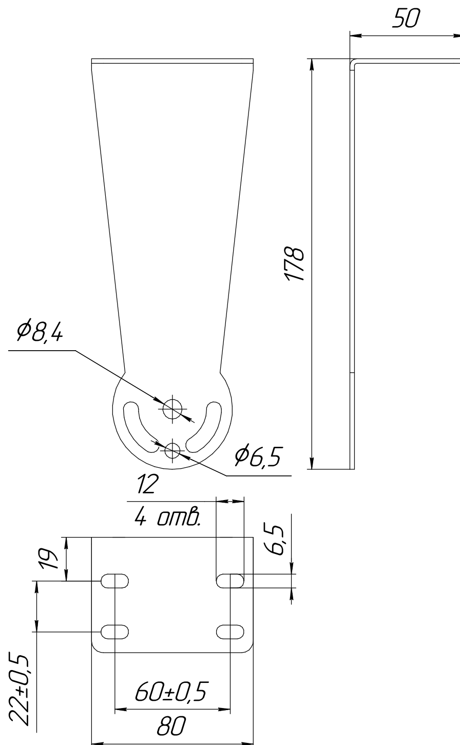
Рисунок 8 - Кронштейн 734313039.
