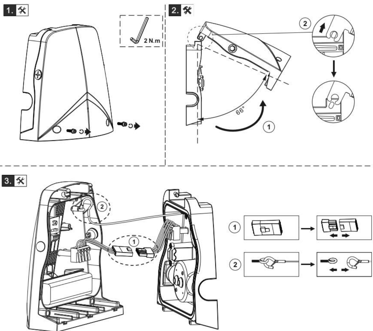
Рисунок 2а - Схема установки светильника.
