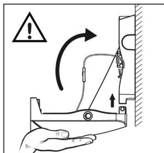
Рисунок 2в - Схема установки светильника.
