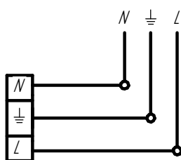
Рисунок 2 - Схема подключения светильника к сети
