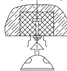
Крепление светильника на опорную поверхность
